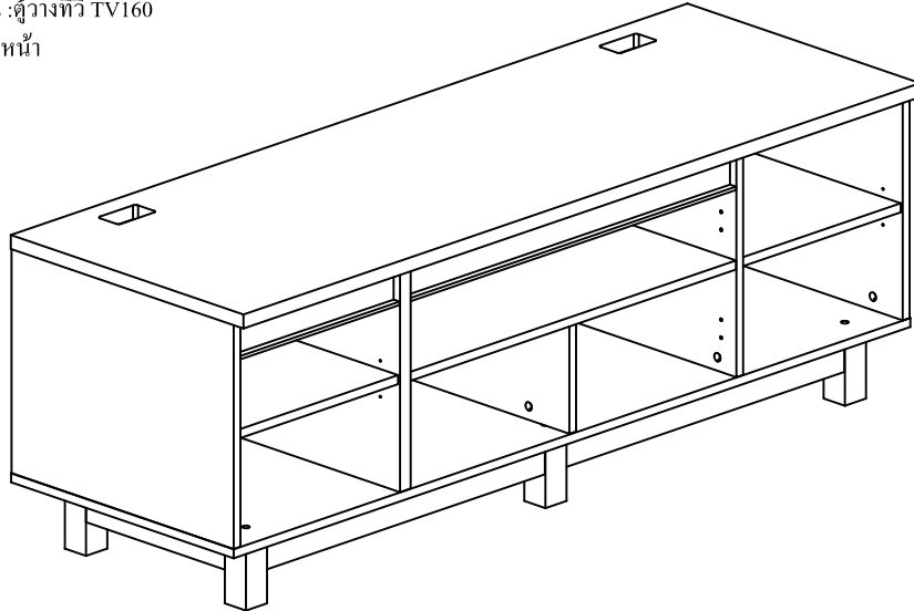
MODEL : ตู้วางทีวี TV160 ภาพด้านหลัง
